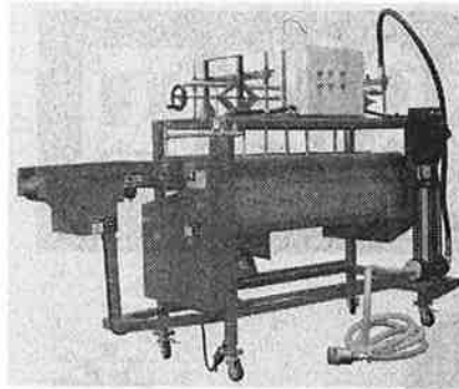
葉付きも洗える大根洗浄機
