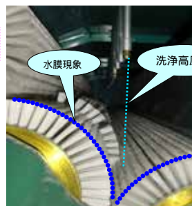
水膜効果イメージ
